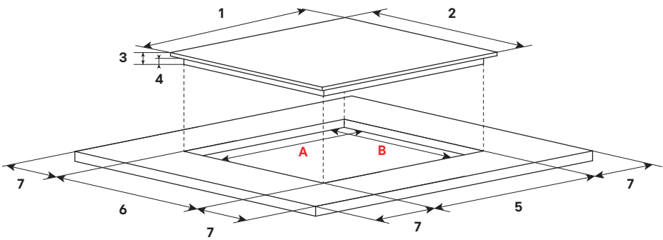
MISURE PER L'INSTALLAZIONE
